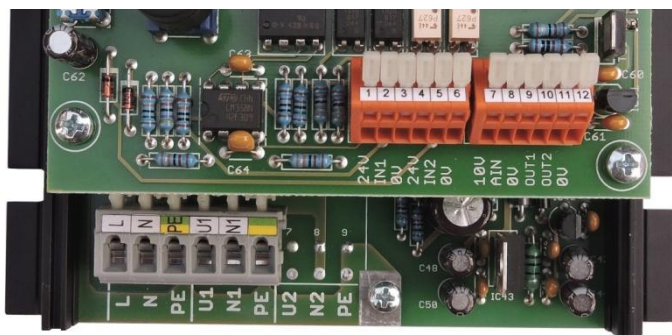
рис. 6 – соединительные зажимы
