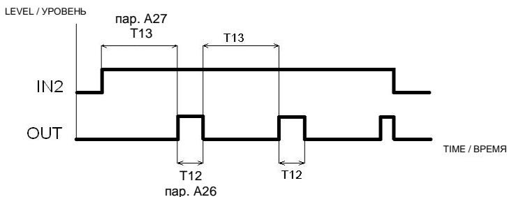
рис. 9b - работа выталкивателя E2
