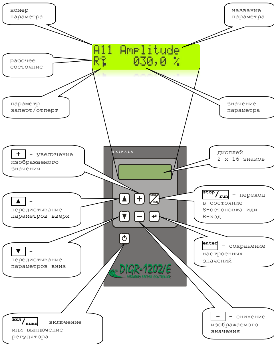
рис. 1 - описание элементов управления
