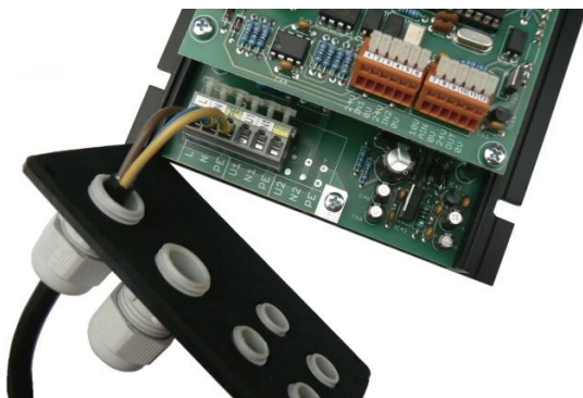
рис. 5 – демонтаж части с выводами
