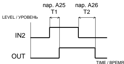
рис. 9а - работа выталкивателя E1
