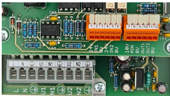
obr. 6 – pripájacie svorky
