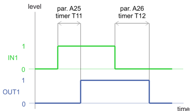
obr. 8 – činnosť vyhadzovača E1
