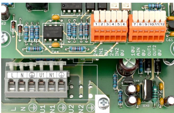
obr. 6 - připojovací svorky
