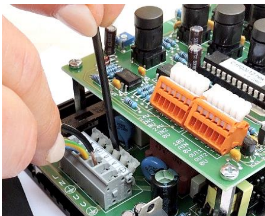
Abb. 7 – Kabelanschluss
