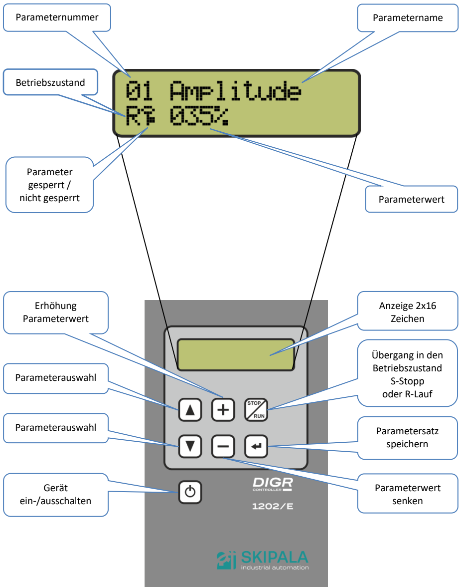
Abb. 1 – Beschreibung Bedienungselemente
