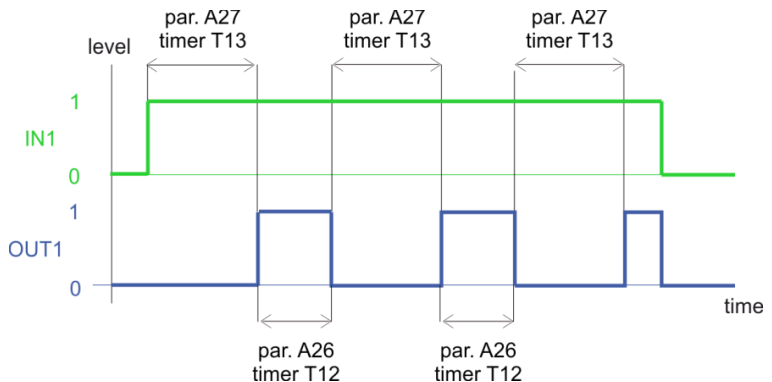
Abb. 9 – Funktionsweise des E2-Auswerfers
