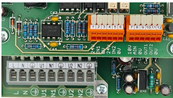
obr. 6 – pripájacie svorky
