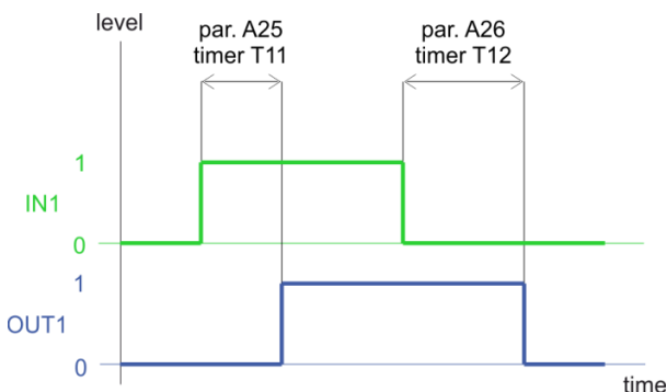
obr. 8 - činnost vyhazovače E1
