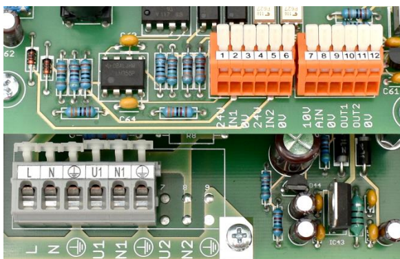
obr. 6 - připojovací svorky
