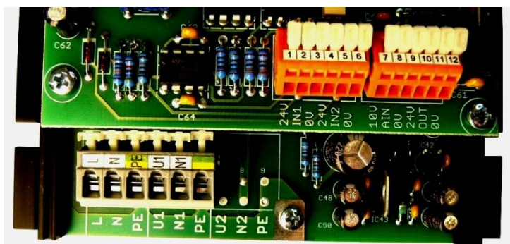
obr. 6 - připojovací svorky
