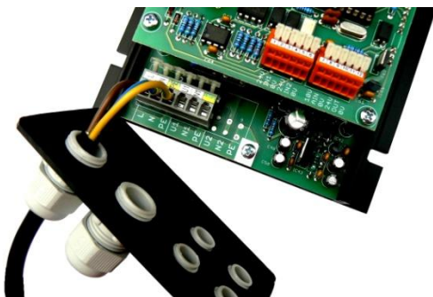
obr. 5 - demontáž části s vývodkami
