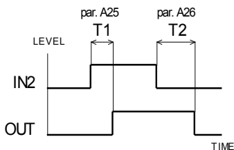
obr. 9 - činnost vyhazovače
