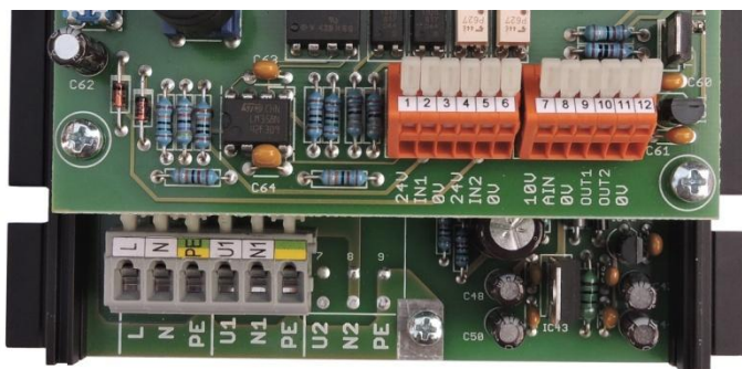
obr. 6 - připojovací svorky
