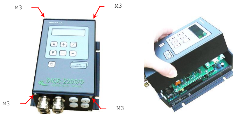
obr. 4 - demontáž víka
