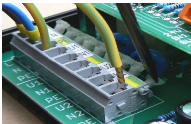
obr. 8 - připojení vodičů do svorek
